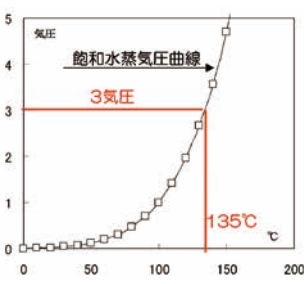
図1 飽和水蒸気圧曲線
