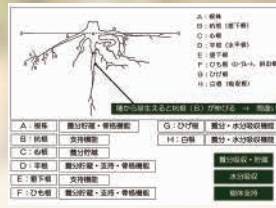
図1 木の根の形
