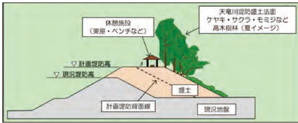
図3 堤防沿い高木樹林ゾーンイメージ断面図
